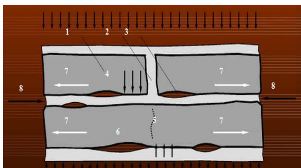
Figura 2. Starea complexă de eforturi în blocuri (cărămizi) și mortar : 1.cărămizi; 2.mortar; 3.goluri de aer;4.zona de compresiune locală;5.secțiune de forfecare; 6. zona încovoiată;7.tensiuni de întindere în cărămizi; 8. tensiuni de compresiune în mortar
