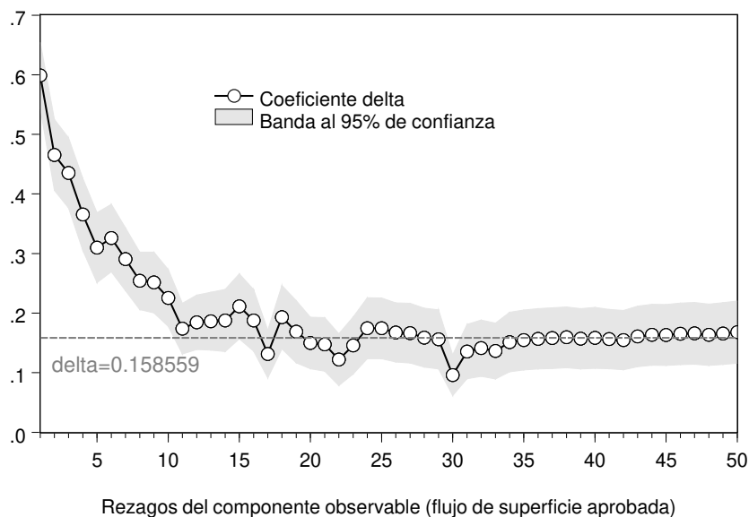
Figura 1: Convergencia del estimador \hat{\delta}_p (tasa mensual de inicios de obra de los permisos habitacionales), según orden del rezago del componente observable (flujo de la superficie otorgada para la edificación de viviendas)
