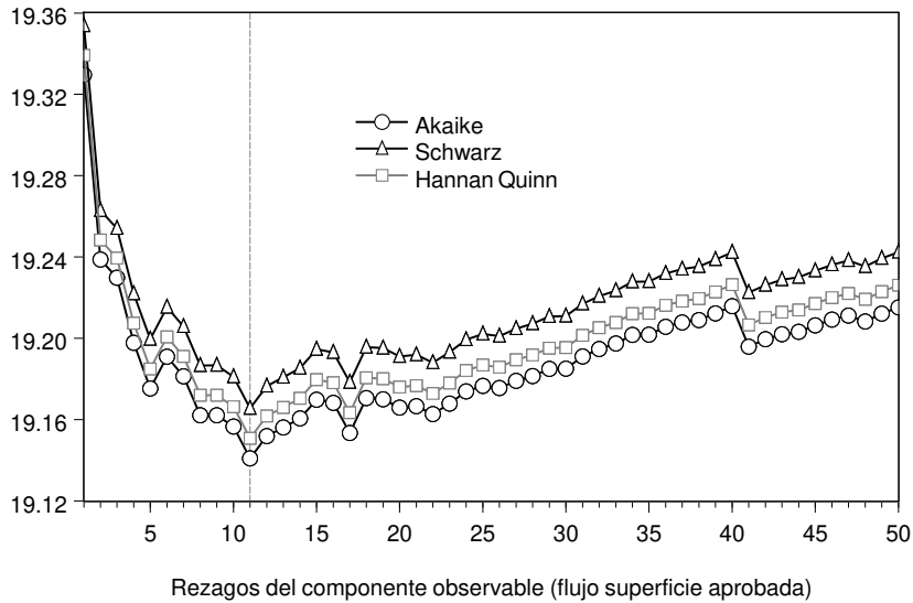
Figura 2: Criterios de información para la selección del orden de rezagos del flujo de permisos de edificación
