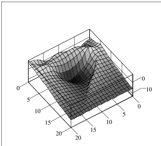
rYL, rYK, rY
