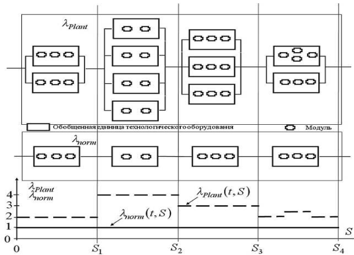
Рисунок 4 – Плотность расположения оборудования \lambda_{norm}(t, S) , \lambda_{Plant}(t, S) , \Delta S_m = 1 .
