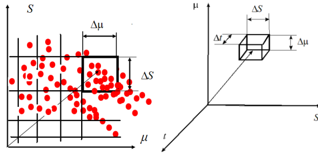
Рисунок 2 – Элементарная ячейка фазового технологического пространства
