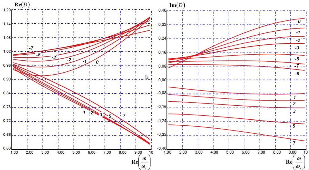
Рис.2. График функции D\left(\varepsilon, \frac{\omega}{\omega_d}\right) для производственной линии ( M=400, v=3, j=2 )
