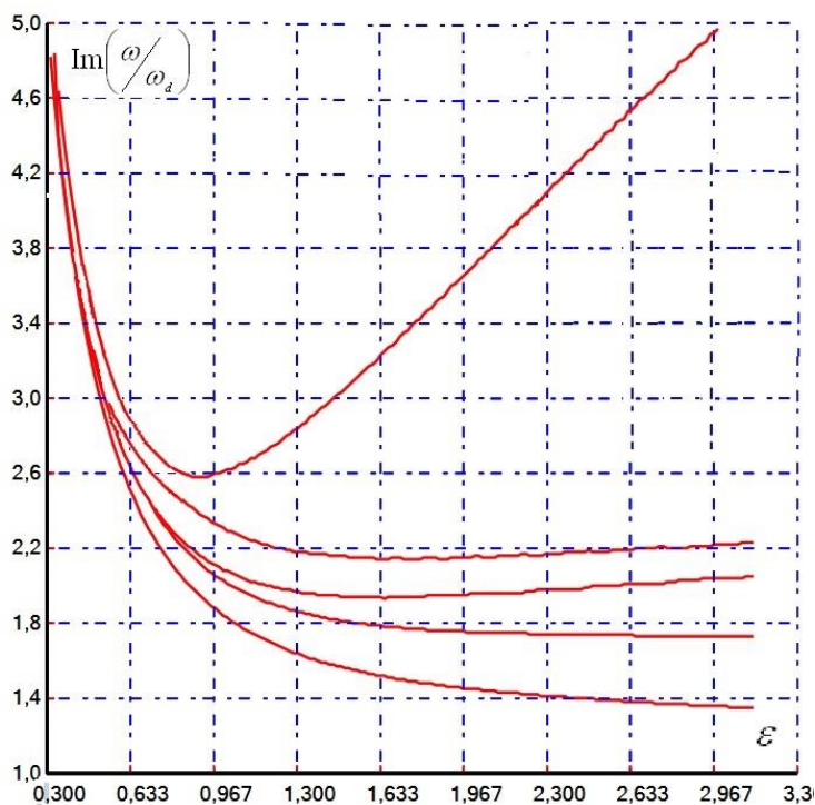
Рис.4. \operatorname{Im} \left( \frac{\omega}{\omega_d} \right) = f(\varepsilon) для производственной линии, \nu=3
